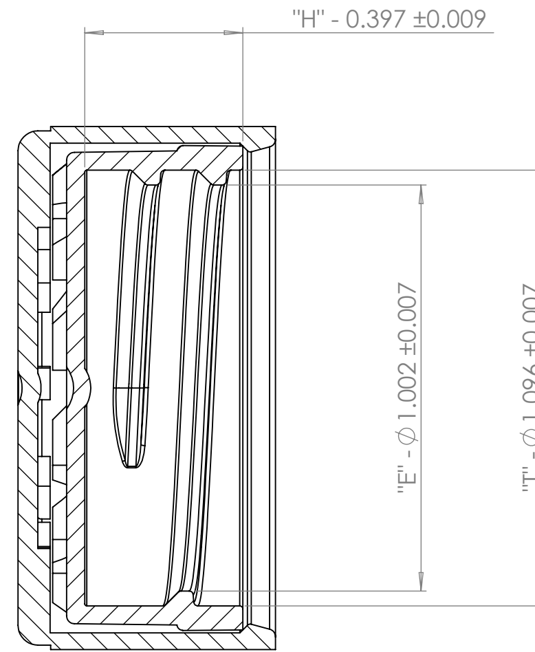
SECTION A-A
